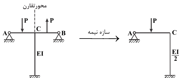
(سازه متقارن تحت اثر بارگذاری پادمتقارن)
