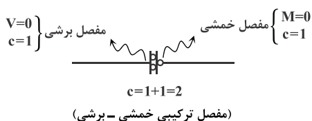
(مفصل ترکیبی خمشی - برشی)
